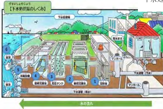
図-3 下水処理のしくみ
